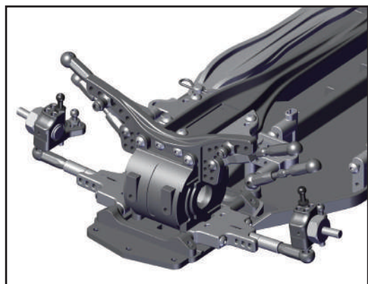
ナックル装着完成図
